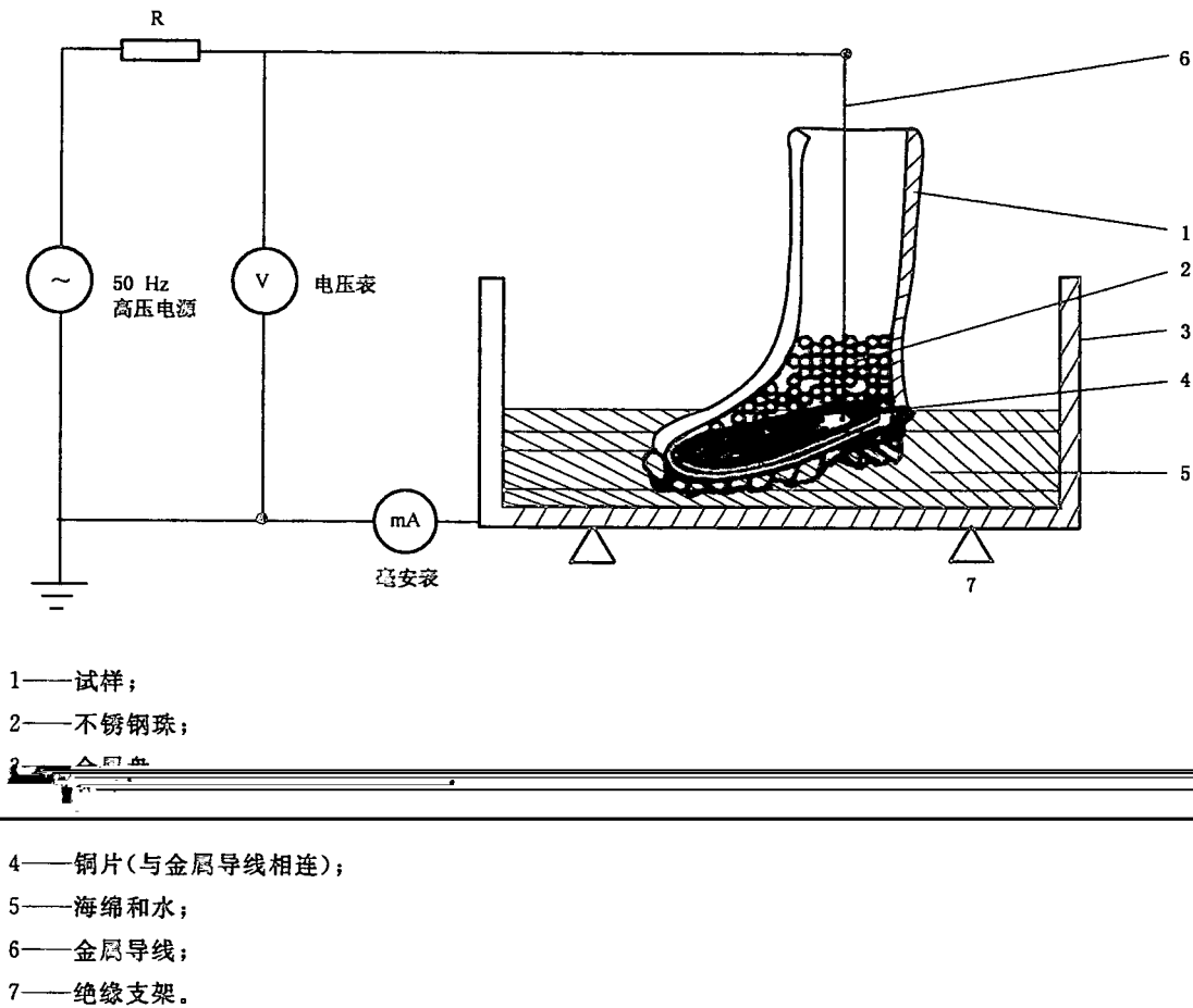
图 3 电绝缘性测试装置
